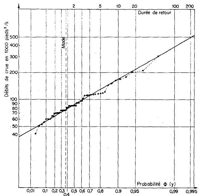
FIG. 6 1 Débits maxima annuels du Colorado à Black Cañon (1878-1929) (Loi de Gumbel)
