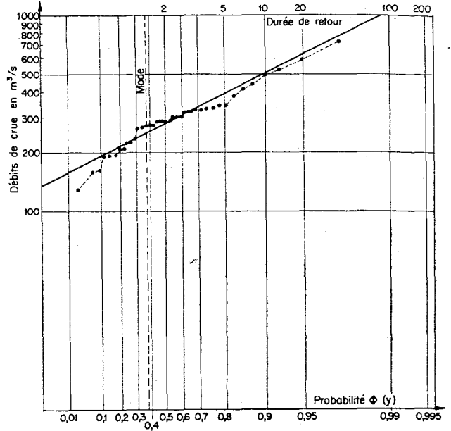
FIG. 7 1 Durance à l'Archidiaere. Crues de printemps 1916-1955 (Loi de Gumbel).
