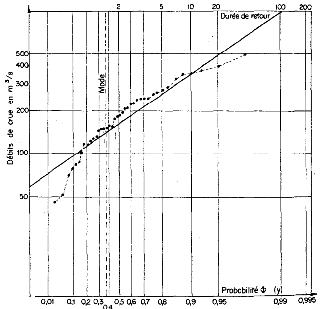
FIG. 8 1 Durance à l'Archidiaere. Crues d'automne 1916-1955 (Loi de Gumbel).
