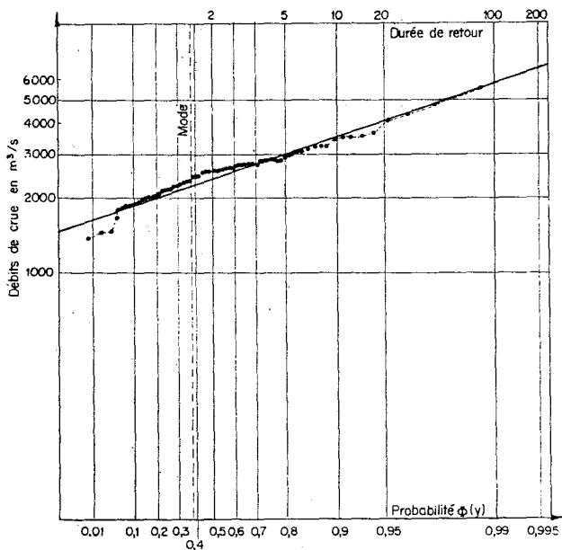
FIG. 5 Débits maxima annuels du Rhin à Rheinfelden (Loi de Fréchet).
