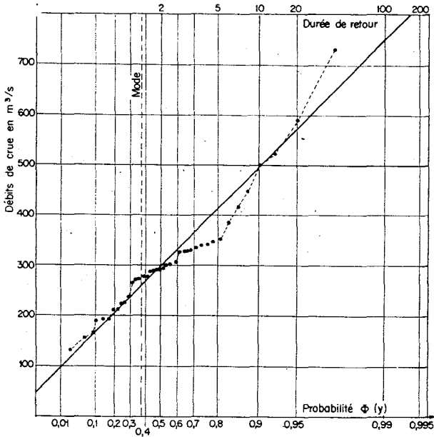
FIG. 7 1 Durance à l'Archidiaere. Crues de printemps 1916-1955 (Loi de Gumbel).
