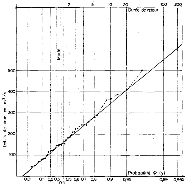
FIG. 8 1 Durance à l'Archidiaere. Crues d'automne 1916-1955 (Loi de Gumbel).
