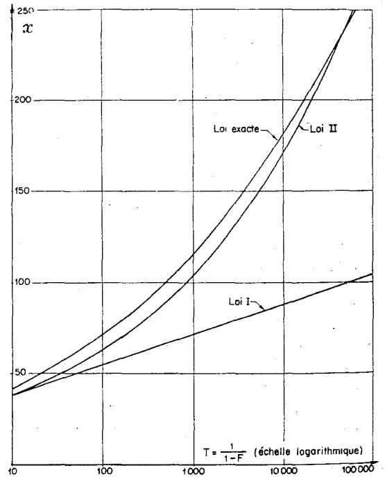
FIG. 3 Loi de la plus grande de 1000 variables galtoniennes. Loi I : F = e^{-e^{-x}} , Loi II : F = e^{-x^{-b}}
