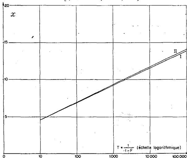
FIG. 2 Loi de la plus grande de 10 variables laplaciennes. I. Loi exacte II. Loi limite
