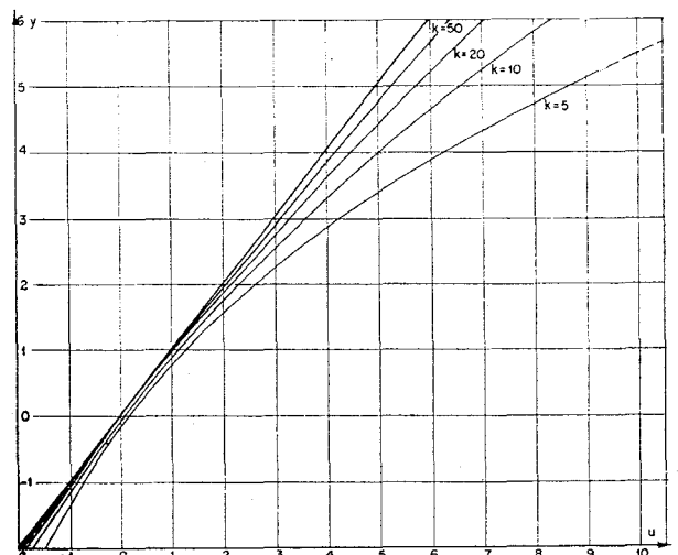
FIG. 4. — Comparaison des lois I : e^{-e^{-y}} et II : e^{-x^{-k}} ou u = k(x - \tilde{x})
